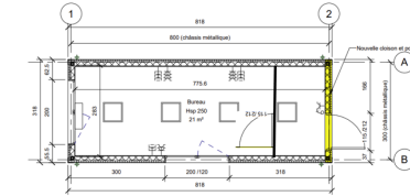
① Vue en plan REZ 1 : 50
